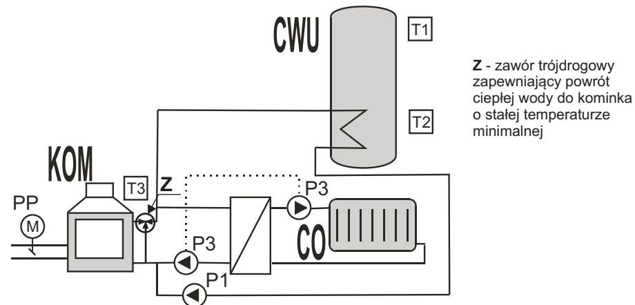
Rys.1b Układ pracy regulatora z wymiennikiem dla obwodu CO (pompa wymiennika i CO podłączone do wyjścia P3)
