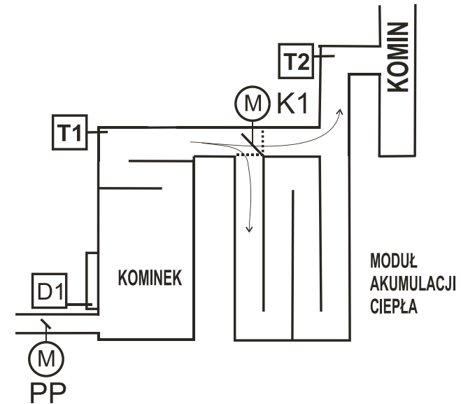
Rys.1 Podstawowy układ pracy regulatora
