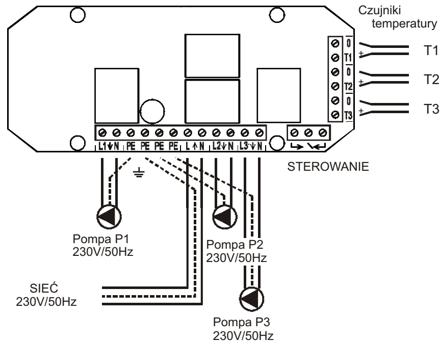
Rys.3 Schemat instalacji elektrycznej
