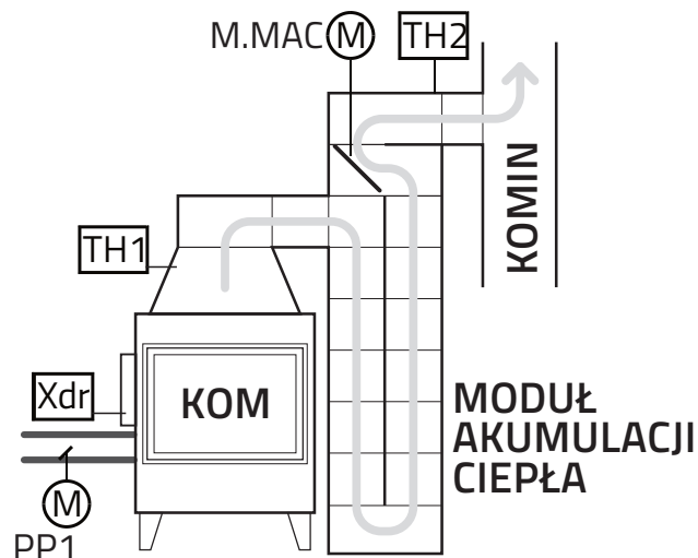
Rys.4 Schemat wykorzystania regulatora do obsługi systemu Modułowej Akumulacji Ciepła (MAC)
