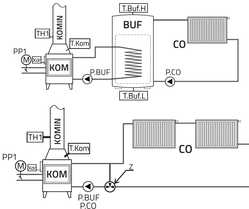
Rys.2 Przykładowe układy pracy regulatora z obsługą nasady/płaszczu wodnego
