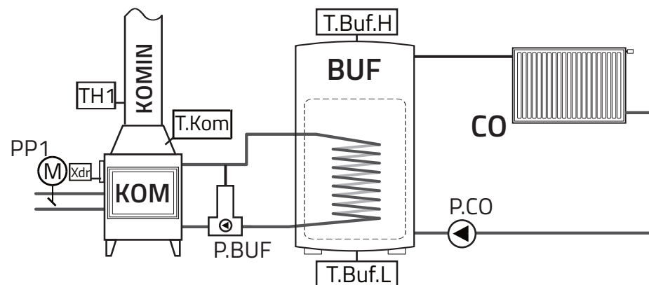
Rys.6 Schemat wykorzystania regulatora do obsługi instalacji wodnej z Laddomatem ładującym bufor ciepła
