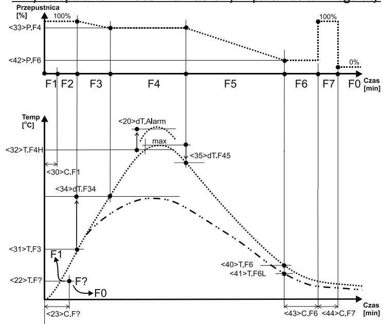
Krzywa spalania RT18os z zaznaczonymi parametrami regulacji
