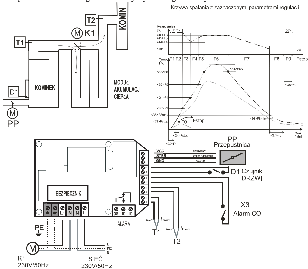
Rys.3 Schemat instalacji elektrycznej
