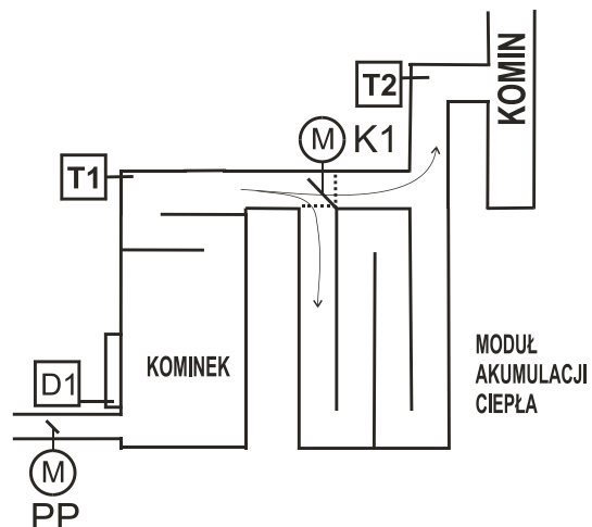
Rys.1 Podstawowy układ pracy regulatora
